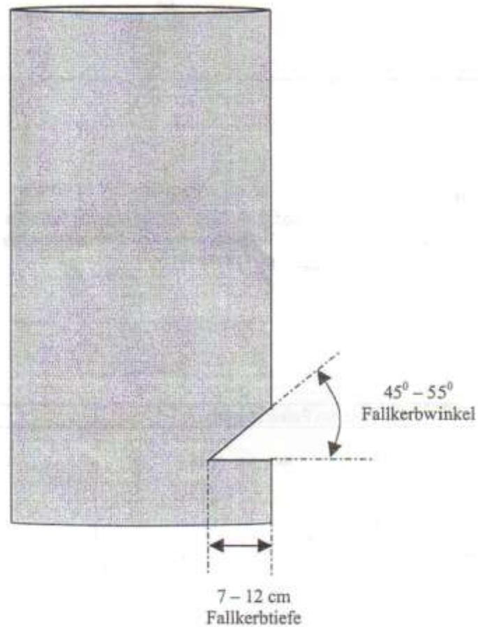
Abb. 13 Fallkerbtiefe / Fallkerbdach
